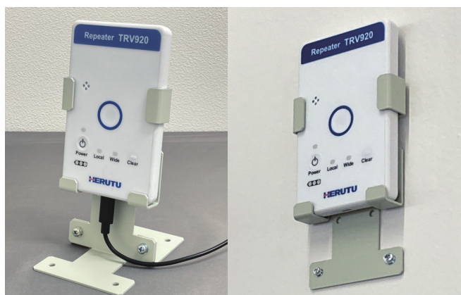
盤上への取付
