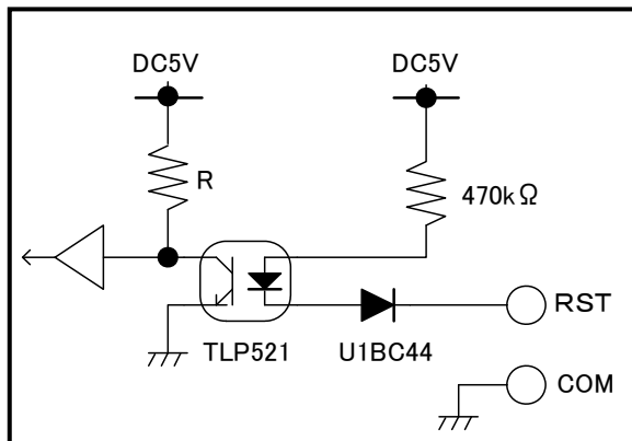
入力回路構成(RST入力)
