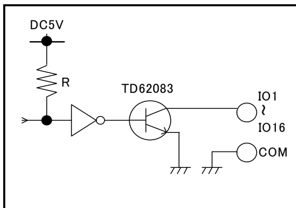
出力回路構成(オープンコレクタ出力)
